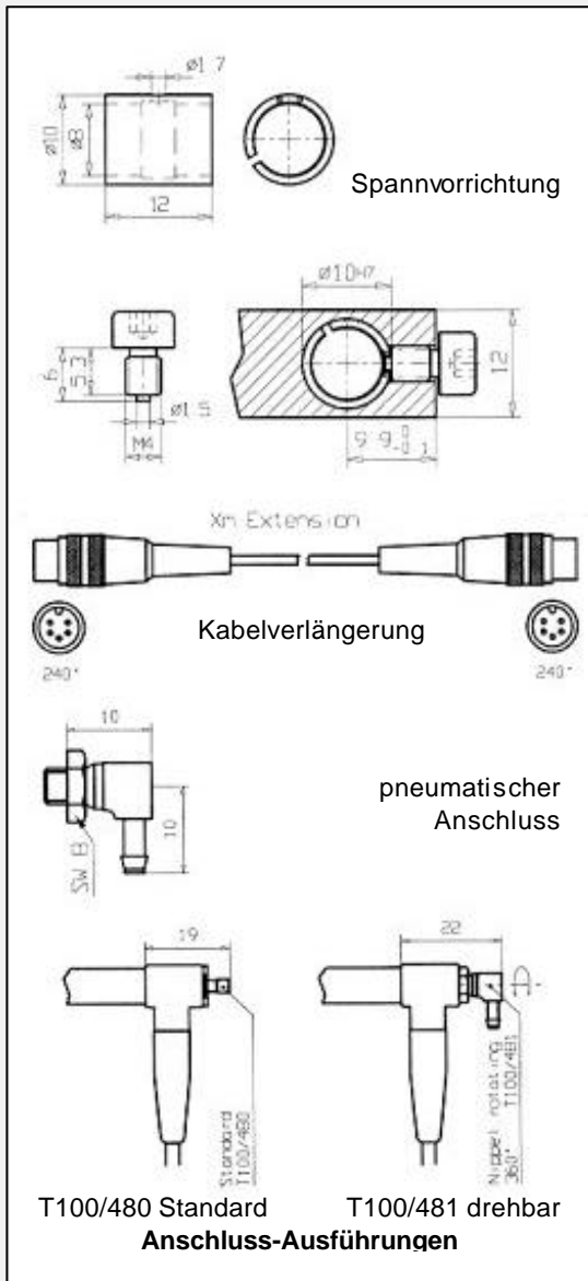
typische Steckeransicht
